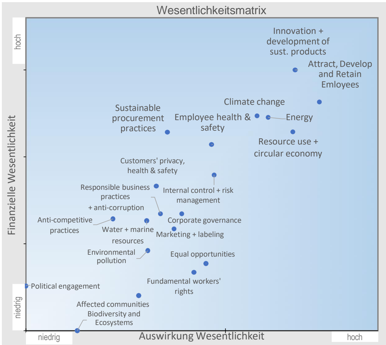
Abbildung 1: Wesentlichkeitsmatrix
